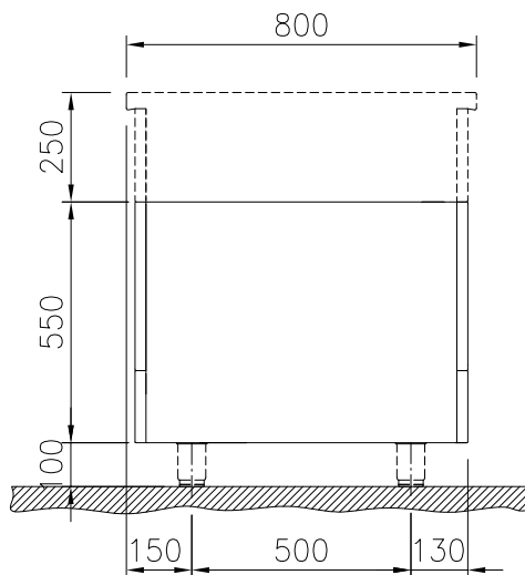
Zij aanzicht
